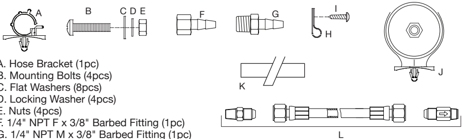
(Fig. 1) 330C-IG 12V / 330C-IG 24V / 450C-IG 12V / 450C-IG 24V Installation Parts List:
